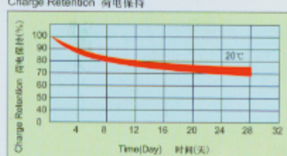
Charge Retention 荷电保持
