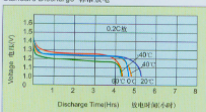
Standard Discharge 标准放电
