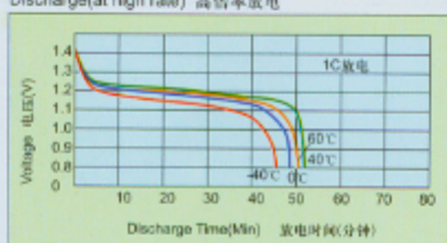
Discharge(at high rate) 高倍率放电
